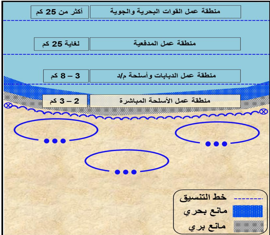
الشكل رقم (5) مناطق عمل الأسلحة
