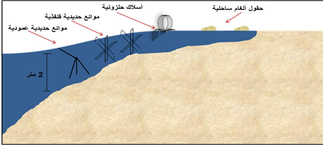
الشكل رقم (4) مقطع عرضي للموانع الساحلية
